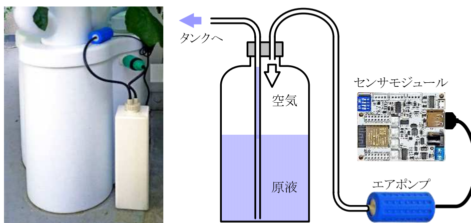
図 6.5 追肥機構
