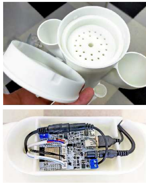
図 6.2 水耕栽培装置のシャワー部とボックス内のセンサモジュール
